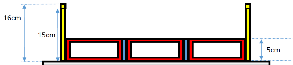
圖二：側視圖
